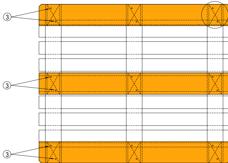
Unteransicht
